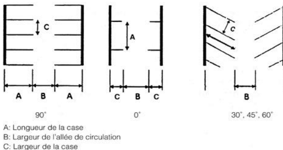
ILLUSTRATION : Dimensions des cases et allées de circulation
